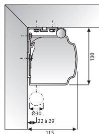
Runder Fallstab
